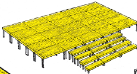
Podestbühne mit vorgebautem breiten 4-stufigen Treppenaufgang.
