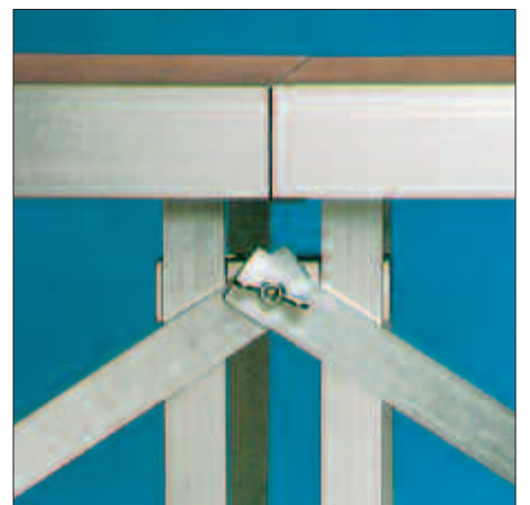
Befestigung von Diagonalstreben, Höhen ab 1,20 m
