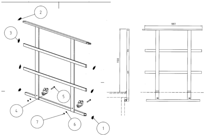
Schutzgeländer für Trenomat FIX/Schere Security rails für Trenomat FIX/Scissor
